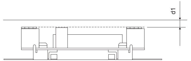
d1=4mm min.
